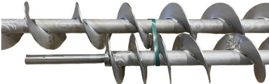
Helsvetsade skruvblad på kärnrör med drivaxel
